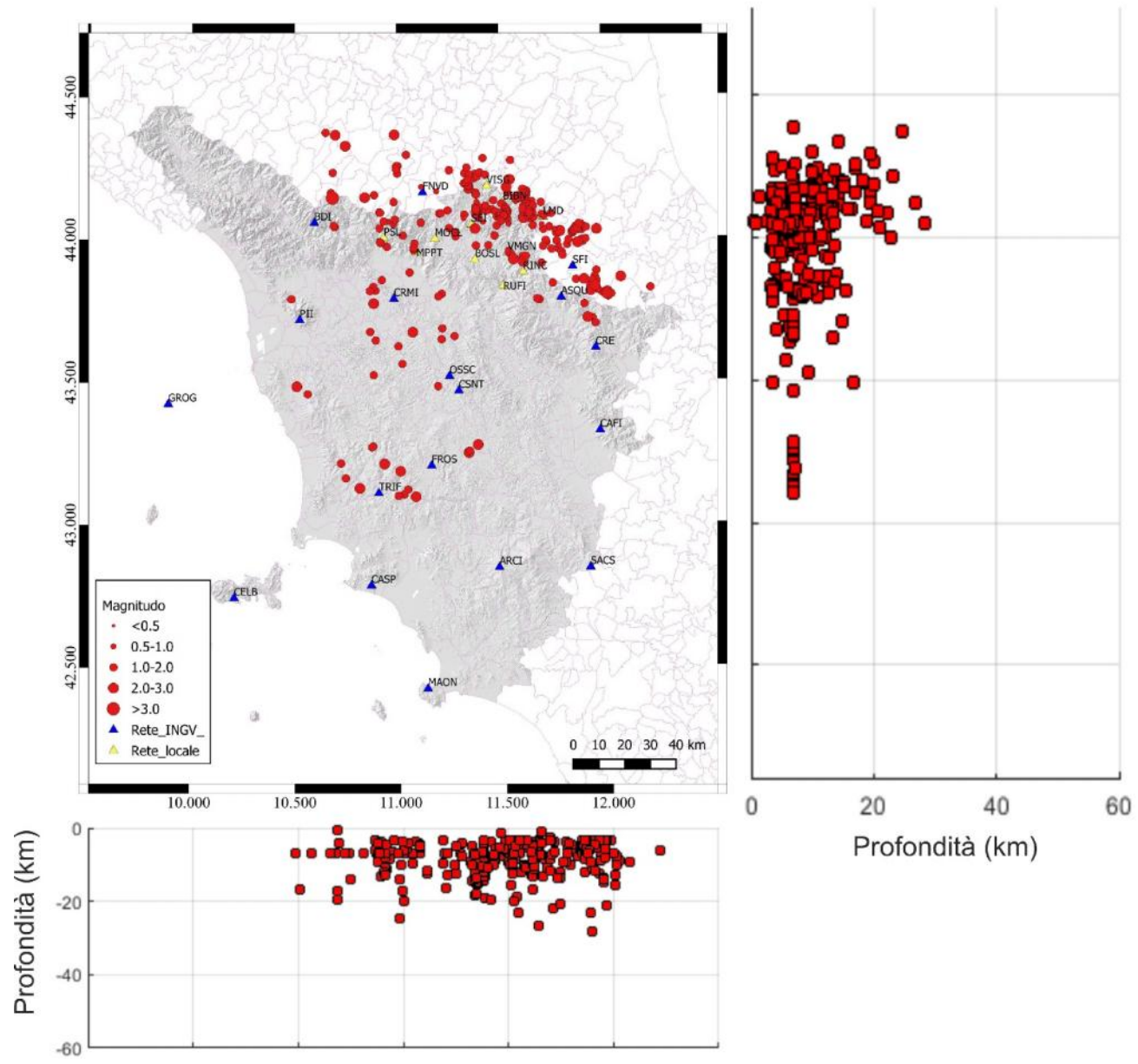
La figura rappresenta la distribuzione della sismicità in Toscana nel corso del 2025. Gli epicentri sono rappresentati da cerchi il cui diametro è proporzionale alla magnitudo, gli ipocentri sono rappresentati tramite sezioni verticali orientate NS e EW allineate con le coordinate della mappa. In generale la sismicità del 2025 ha mantenuto caratteristiche simili a quella del 2024 con sismicità diffusa nelle aree appenniniche e alcune sequenze arealmente ristrette come quella di Palazzuolo sul Senio (21 eventi M_l(\max)=2.5 ). Complessivamente il numero di eventi è stato minore.
